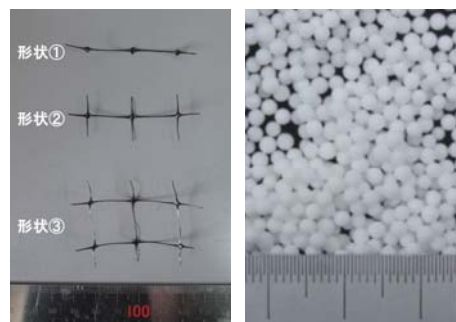
混入させている材料 (左：発泡ビーズ、右：短繊維)
